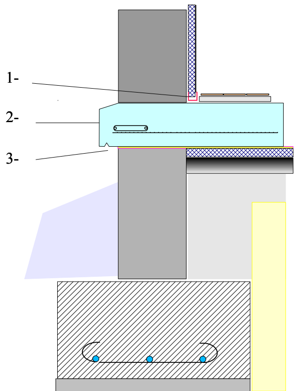
1 U Plastique 2 Profil de rive saillant en forme de larmier 3 Film étanche 200 microns
